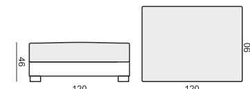
FOOTSTOOL 120x90
