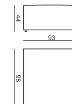
FOOTSTOOL 93x98
