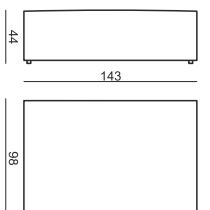
FOOTSTOOL 143x98
